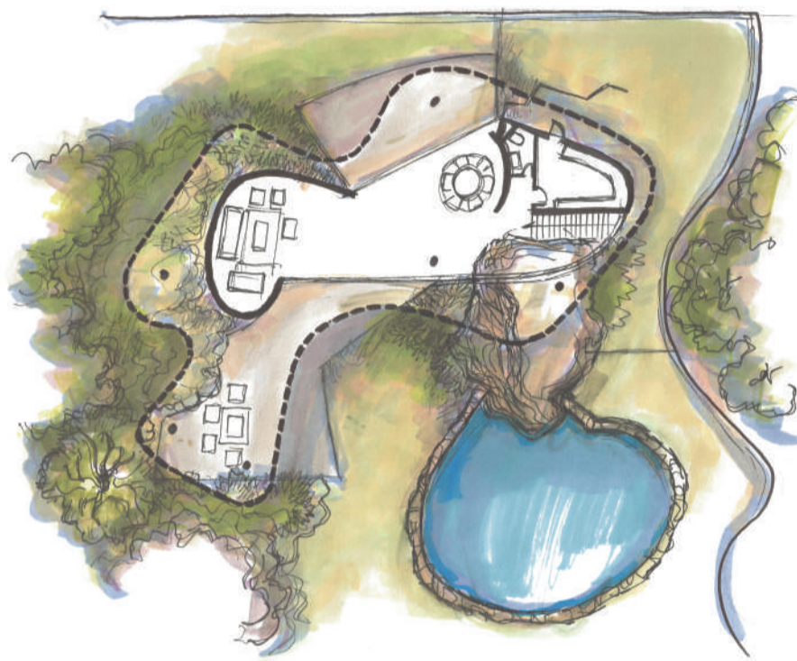
OSCAR NIEMEYER /// VILLA CANOAS /// ENVIRON DE RIO (BARRA DE TIJUCA) /// 1951
